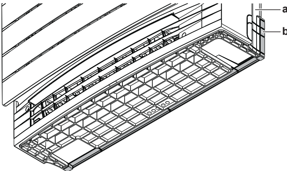
a Bâti inférieur b Partie fendue
