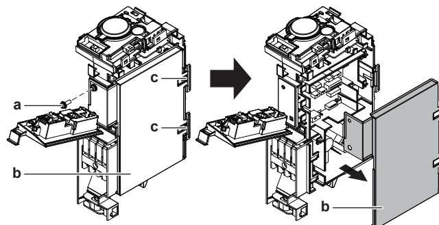
a Vis b Couvercle du coffret de câblage c Languettes
