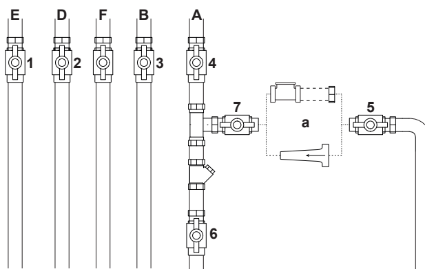
a Utilisez un sectionneur ou un double clapet anti-retour conformément aux réglementations locales.
