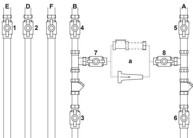
a Utilisez un sectionneur ou un double clapet anti-retour conformément aux réglementations locales.
