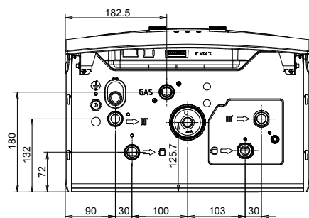
Vue de dessous des modèles D2TND028A4AB et D2TND035A4AB
