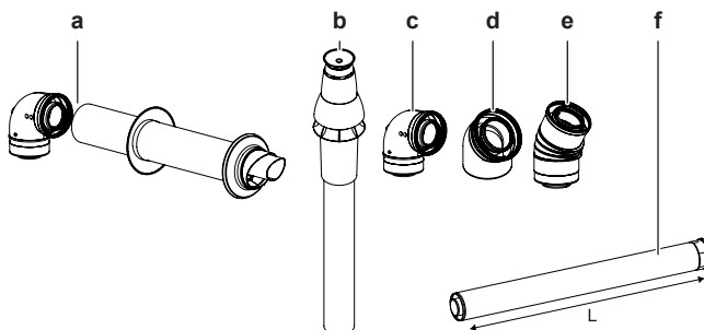
a Adaptateur 60/100 vers 80/125
