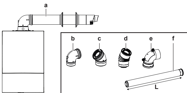
a Kit de terminal pour mur 60/100
