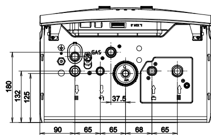
Vue de dessous des modèles D2CND028A4AB et D2CND035A4AB
