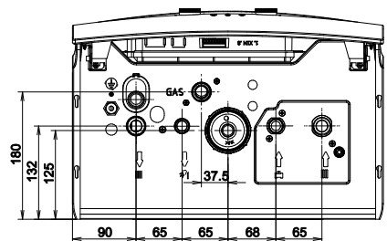
Vue de dessous des modèles D2TND028A4AB et D2TND035A4AB
