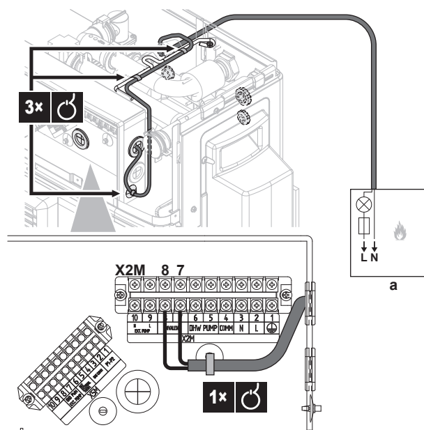
a Signal relève pour chaudière à gaz tierce
