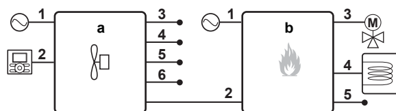
a Unité extérieure b Chaudière à gaz EHY2KOMB28+32AA
