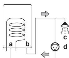
a Raccord de recirculation b Raccordement d'eau chaude
