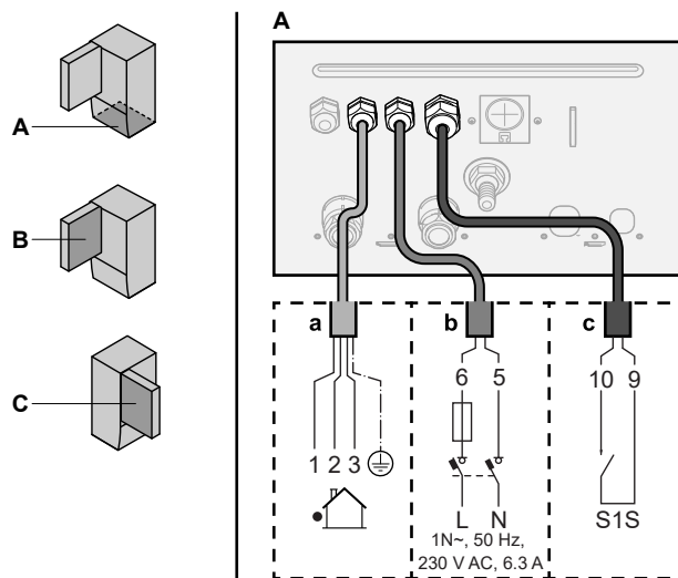
a Câble d'interconnexion (=alimentation électrique principale) b Alimentation électrique à tarif normal c Contact d'alimentation électrique préférentielle
