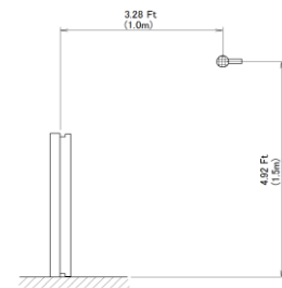
Emplacement de mesure (côté évacuation)
