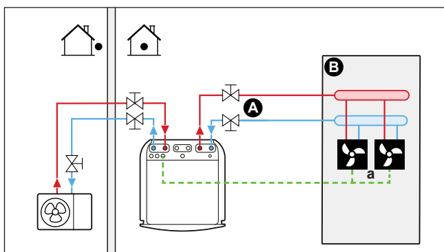
A Zone de température de départ principale
