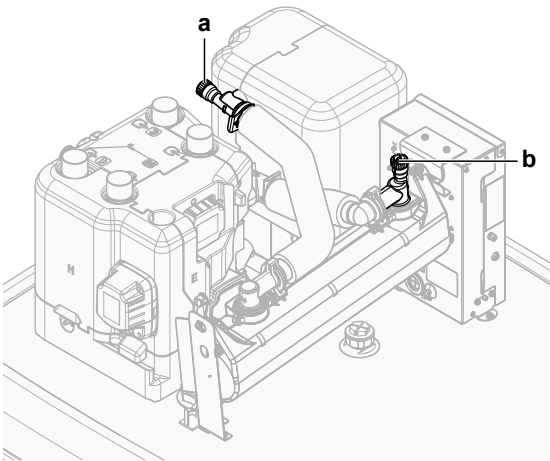
a, b Vanne de purgeur d'air manuelle
