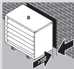
a Couvercle à réduction sonore
