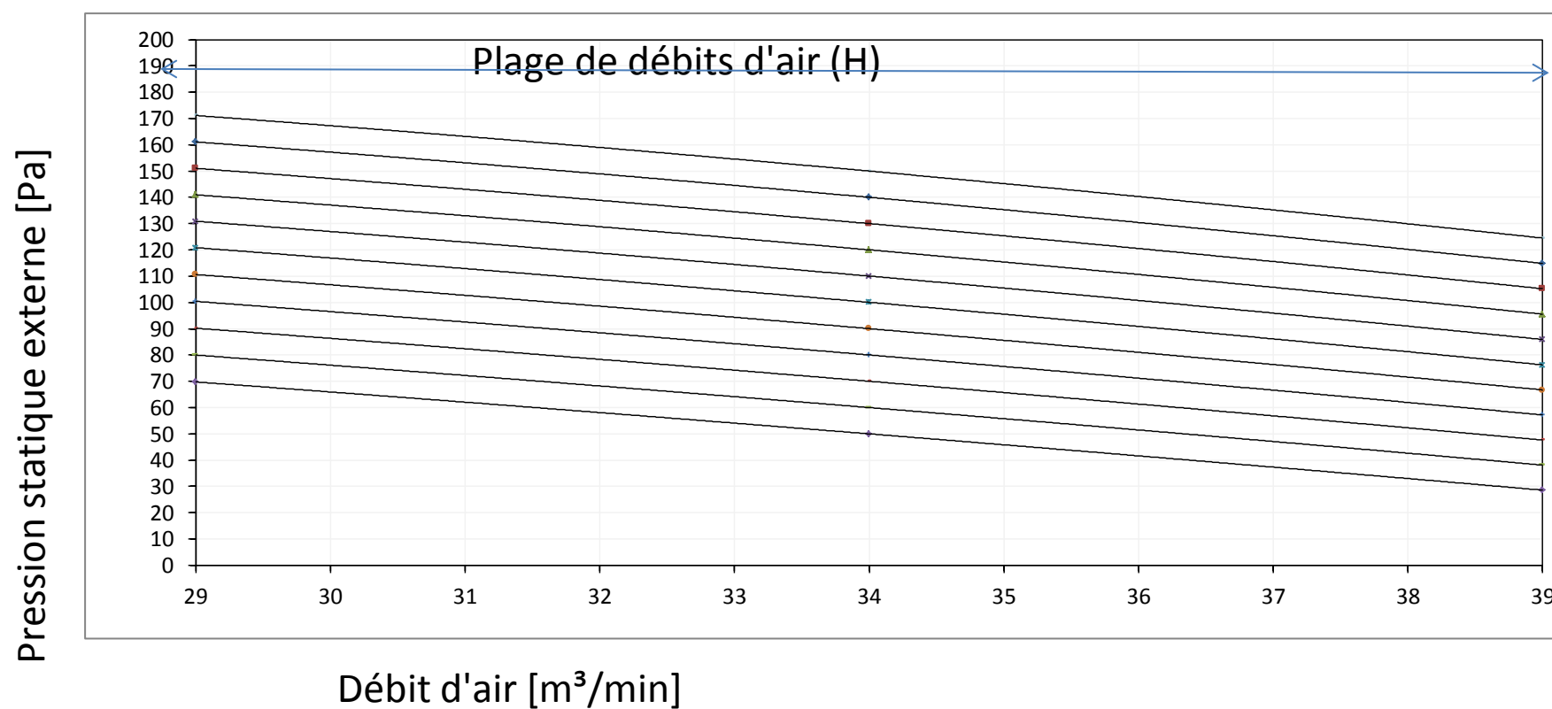
Caractéristiques du ventilateur (2) Réglage sur place avec la télécommande
