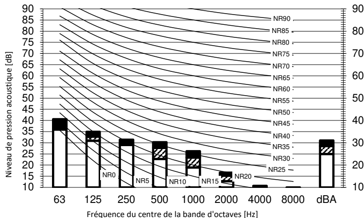
Mode rafraîchissement
