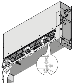
aspiration par l'avant
