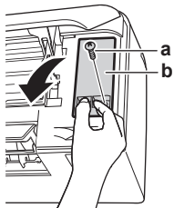
a Vis du couvercle d'entretien b Couvercle d'entretien
