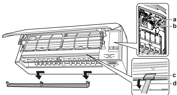
a Connecteur b Attache c Couvercle de vis d Longue plaque plate enveloppée dans un chiffon
