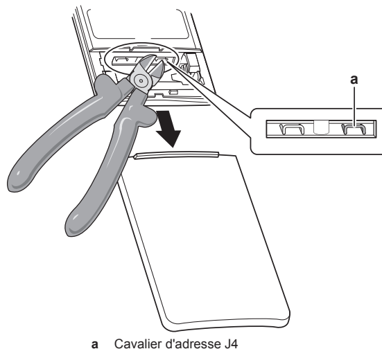
a Cavalier d'adresse J4
