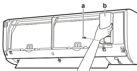
a Vis du couvercle d'entretien
