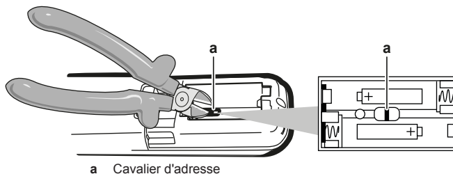
a Cavalier d'adresse
