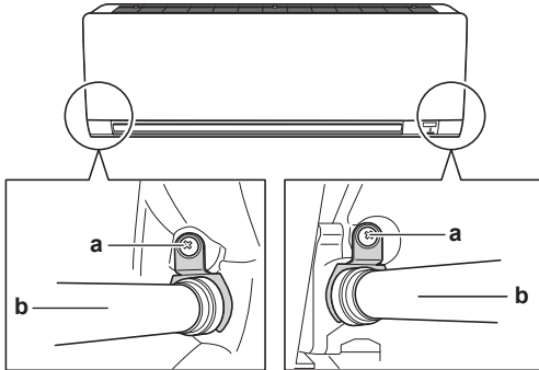
a Vis de fixation d'isolation b Tuyau de purge
