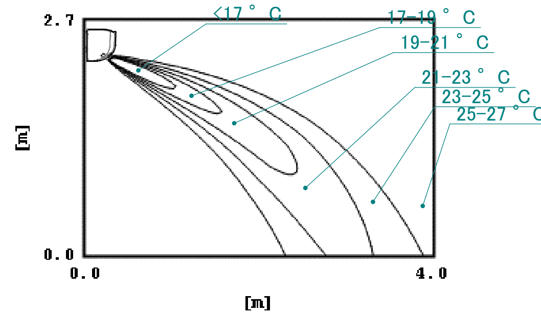
Répartition de la température ambiante (chauffage) Sens du flux d'air: vertical
