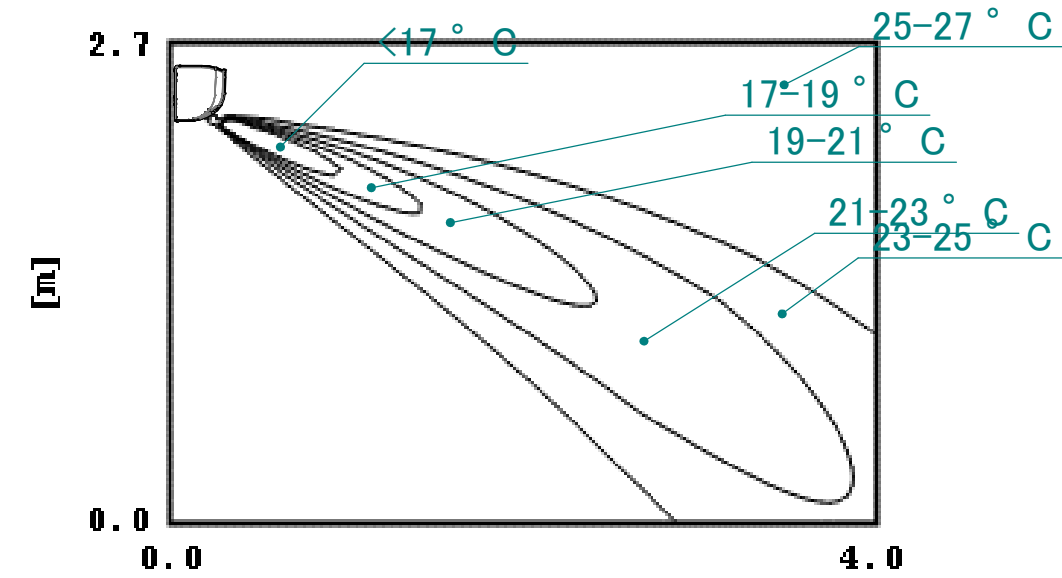
Répartition de la température ambiante (rafraîchissement) Sens du flux d'air: horizontal
