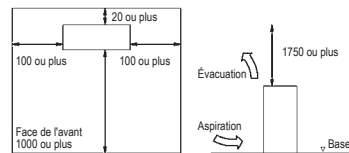
Espace d'installation requis
