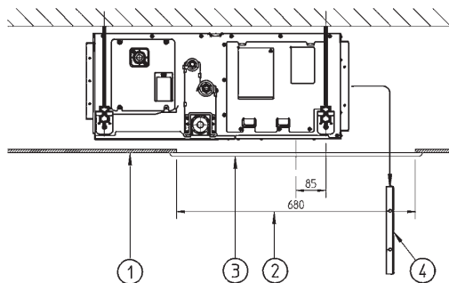
Installation sans conduite de prise d'air
