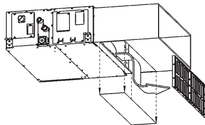
Installation avec conduite de prise d'air
