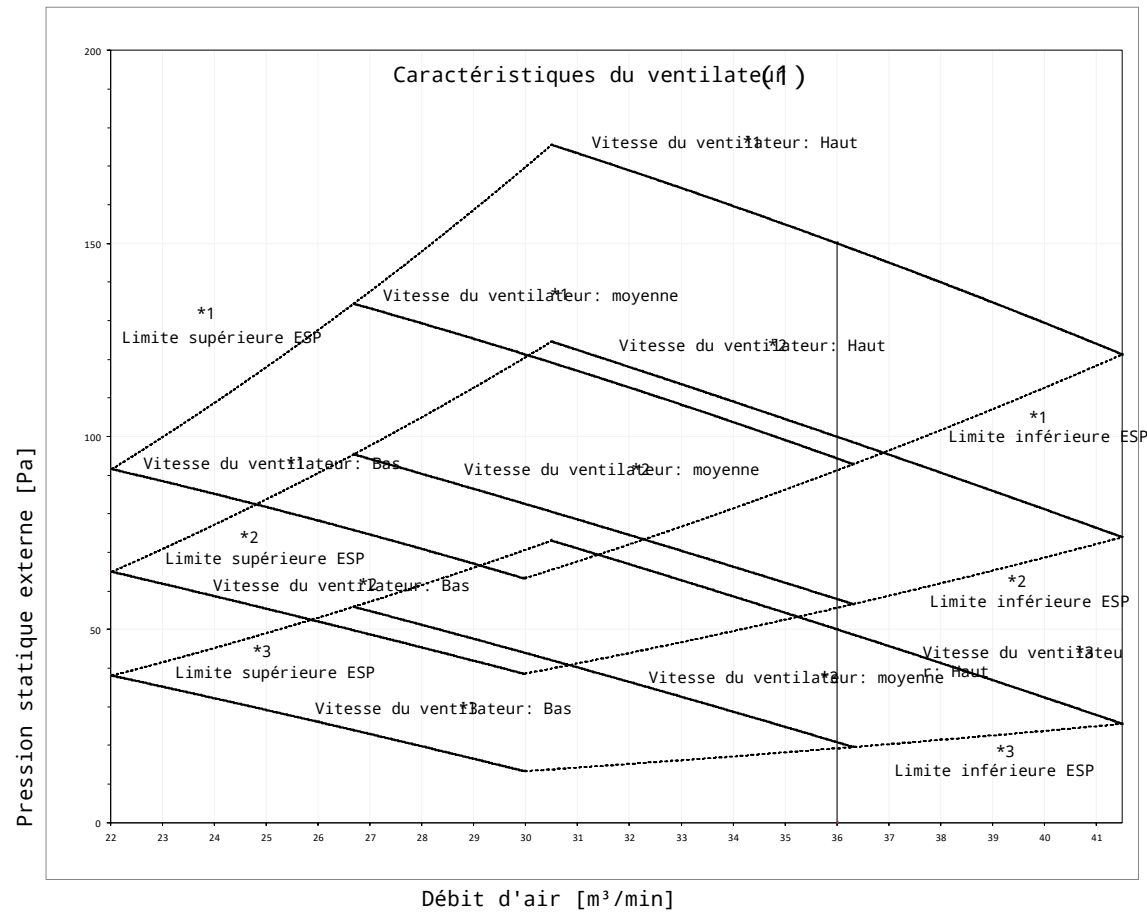
Caractéristiques du ventilateur (c) Réglage sur place avec la télécommande
