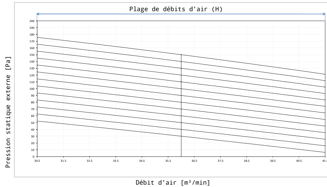
Caractéristiques du ventilateur (c) Réglage sur place avec la télécommande
