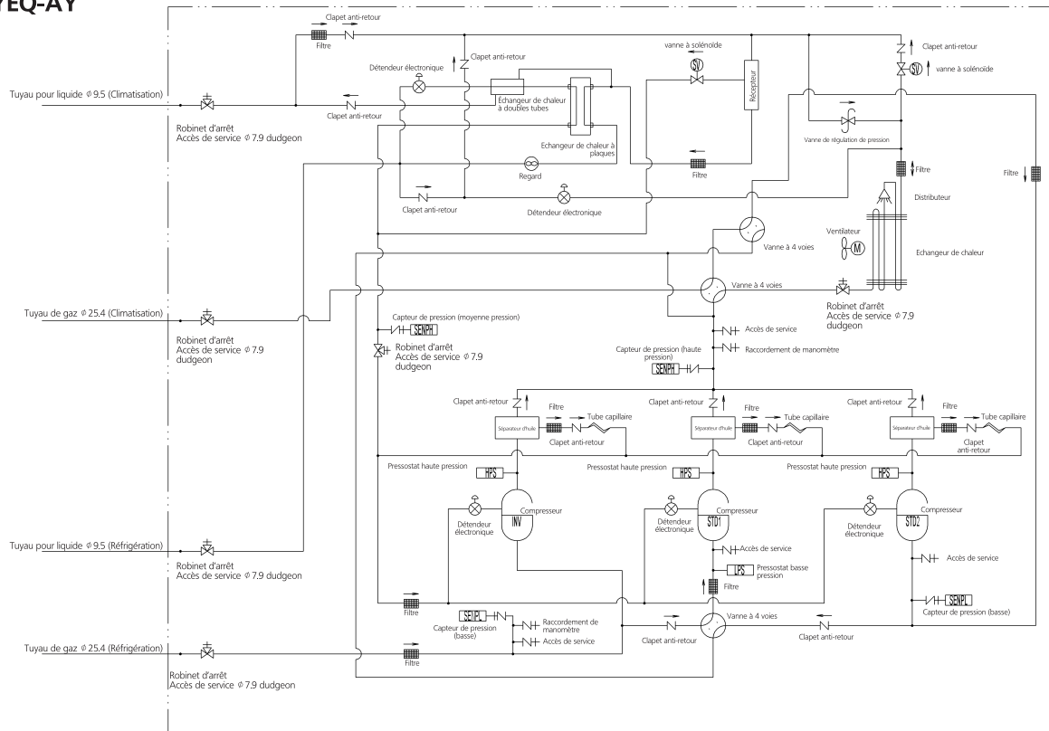
Unité extérieure
