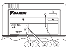
① ② clignotent ③ lampe témoin (allumée)
