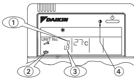
(2) Pendant la vérification du fonctionnement
