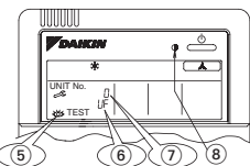
① ② ③ ⑤ ⑥ ⑦ clignotent Lampes témoins ④ ⑧ (clignotent)
