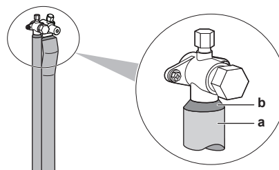
a Matériau d'isolation b Matage, etc.
