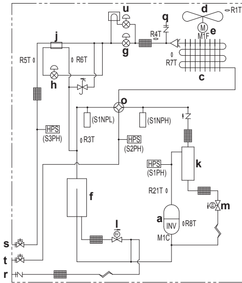
Schéma de tuyauterie: RXYQQ8~12
