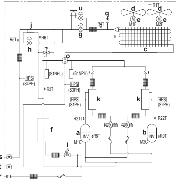
Schéma de tuyauterie: RXYQQ14~20
