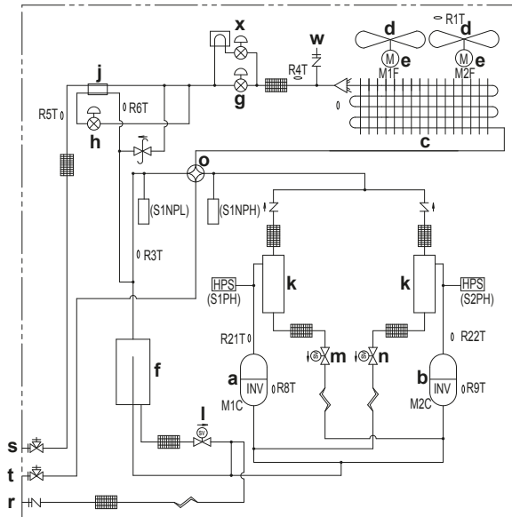
Schéma de tuyauterie: RXYQ14~20
