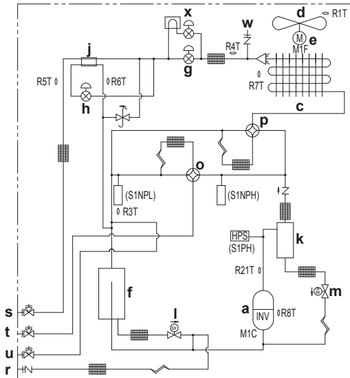
Schéma de tuyauterie: RYMQ8~12
