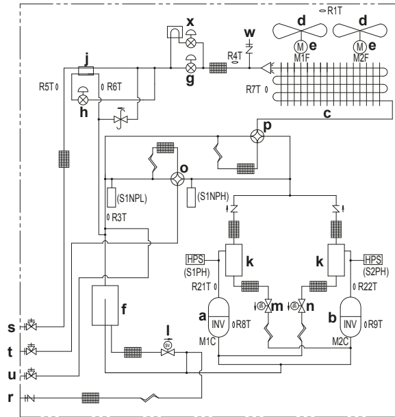
Schéma de tuyauterie: RYMQ14~20
