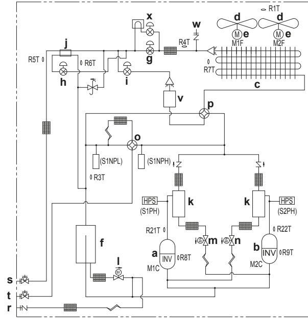
Schéma de tuyauterie: RYYQ14~20
