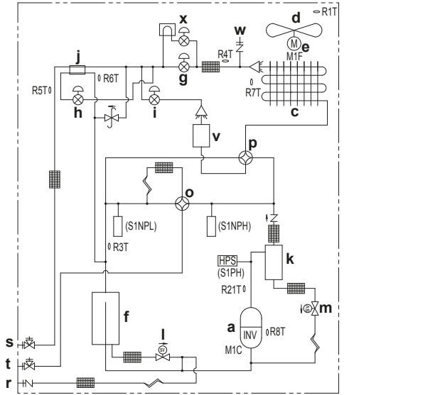
Schéma de tuyauterie: RYYQ8~12
