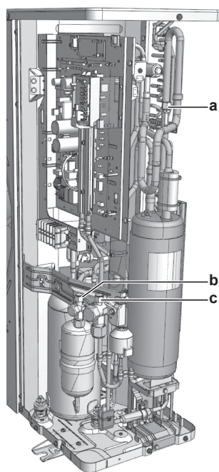
RZQG71_Y1 + RZQSG100+125_Y1
