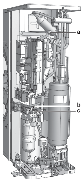
RZQG71_Y1 + RZQSG100+125_Y1
