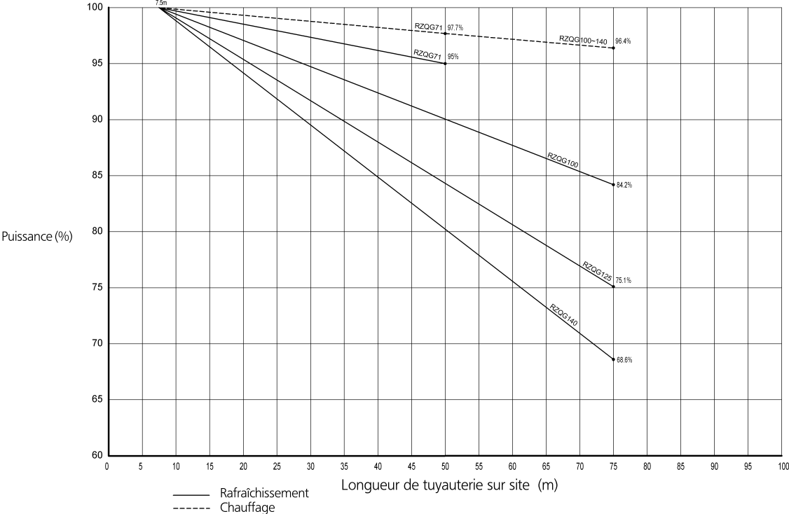
Puissance en fonction de la longueur de tuyauterie sur site pour système avec inverter
