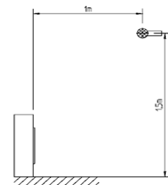
Emplacement de mesure (côté évacuation)
