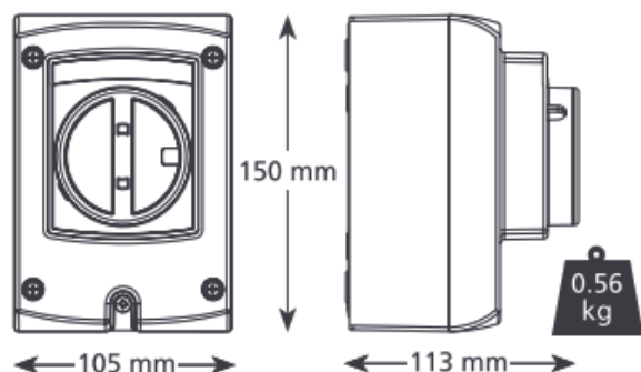
modèle 20 A / 32 A
