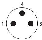
Schéma des pôles, connecteur mâle M8, 3 pôles, vue côté mâle
