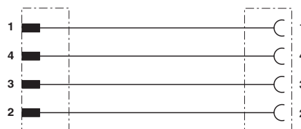
Disposition des contact des connecteurs mâles/femelles M8
