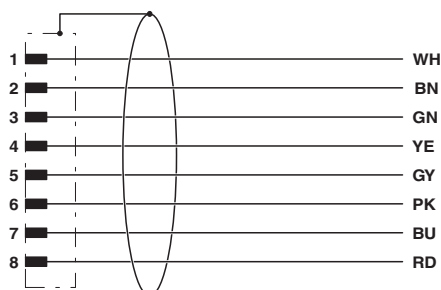
Affectation des contacts des connecteurs mâles M12
