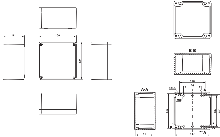
Dessin coté
