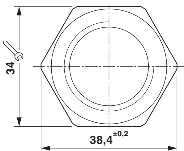
Dessin coté
