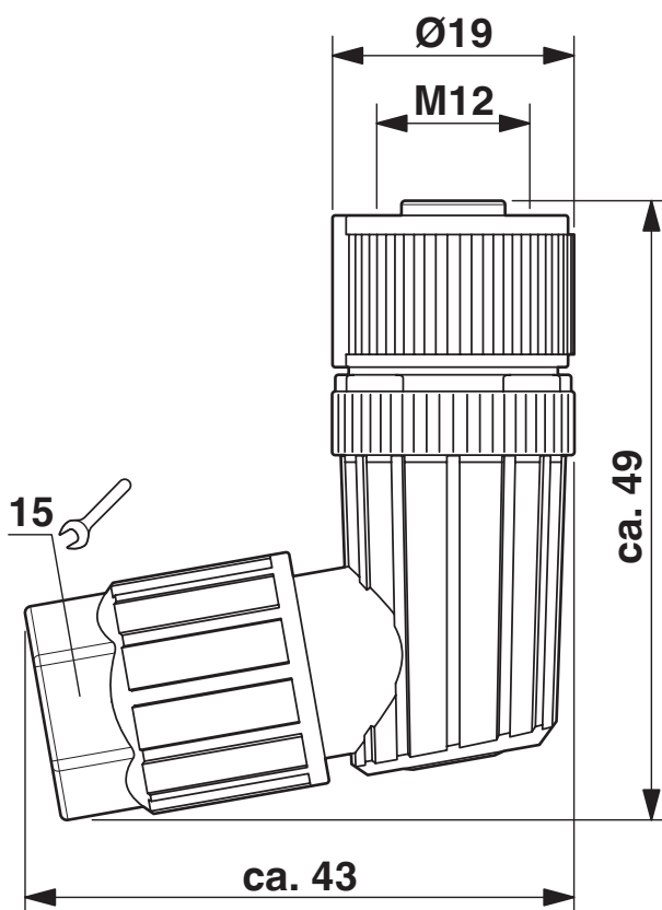
Dessin coté
