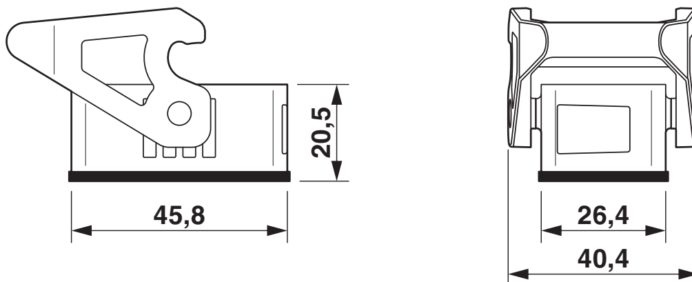
Dessin coté
