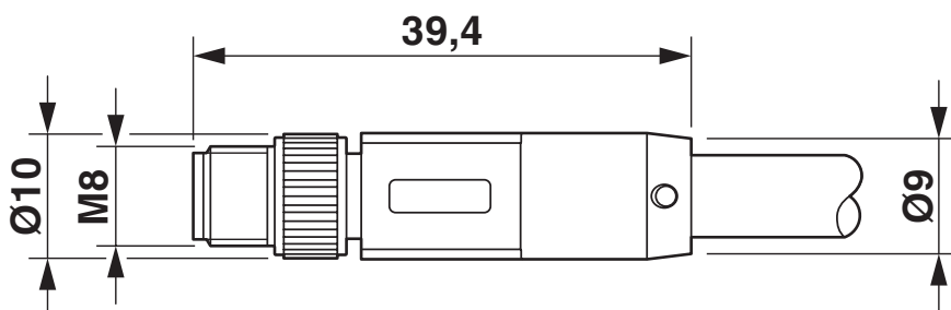
Dessin coté
