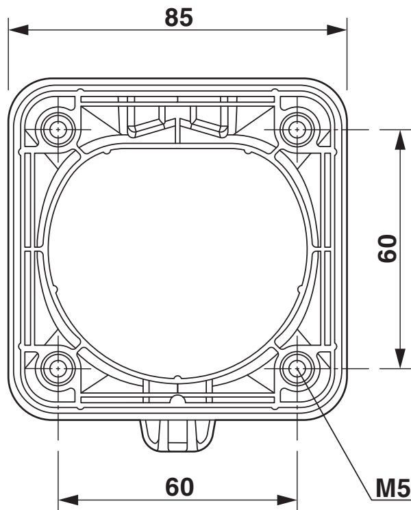
Dessin coté
