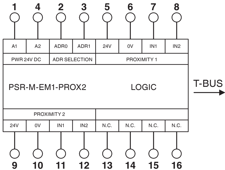
Schéma fonctionnel
