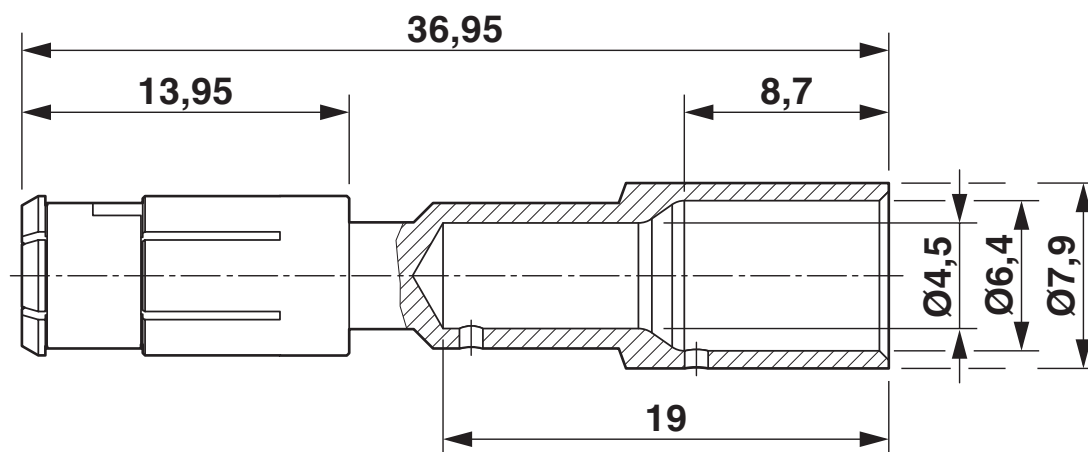
Dessin coté
