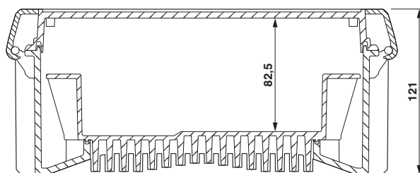
Dessin coté
