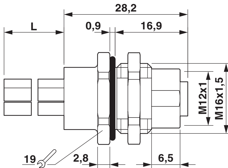
Dessin coté
