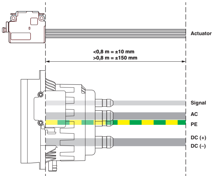
Dessin coté
