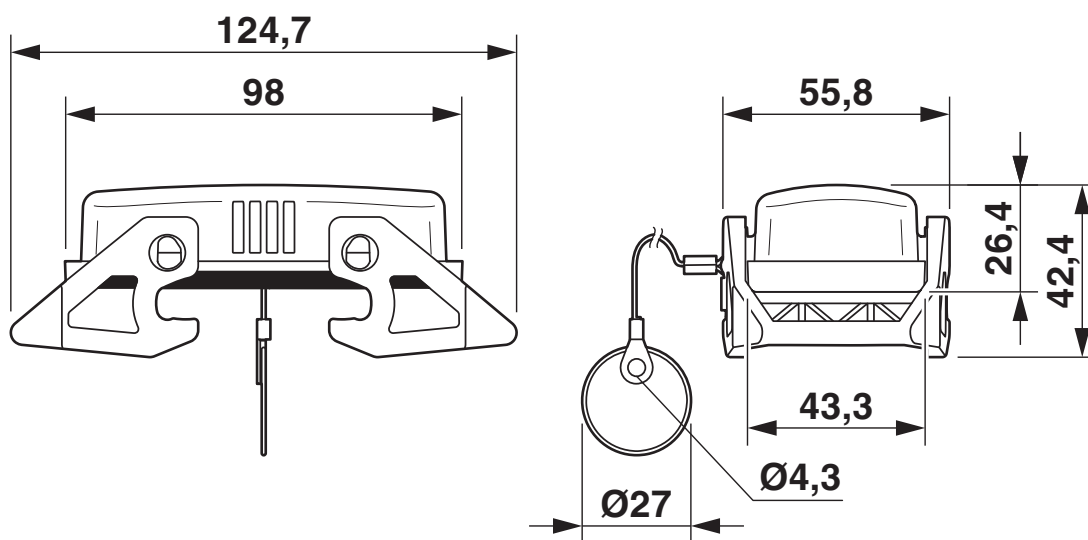
Dessin coté
