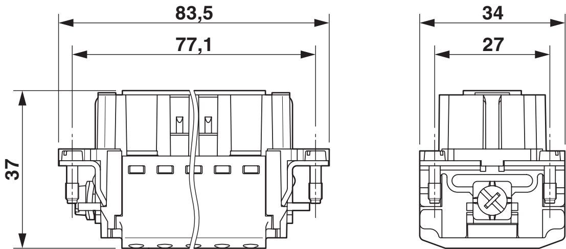
Dessin coté
