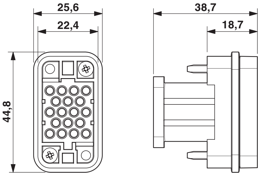
Dessin coté
