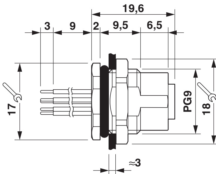
Dessin coté
