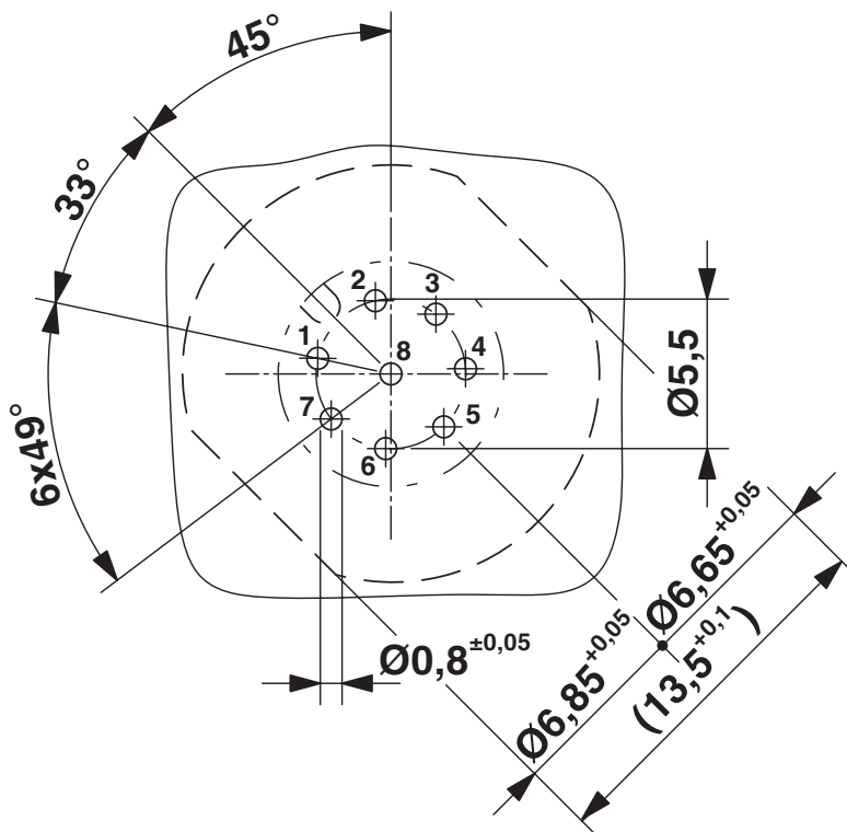
Gabarit perçage / géom. pastille soudage
