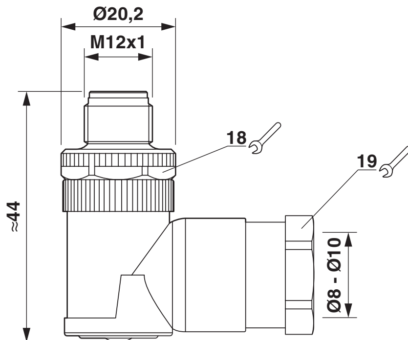
Dessin coté
