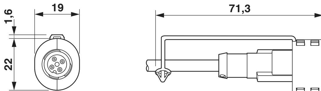
Dessin coté
