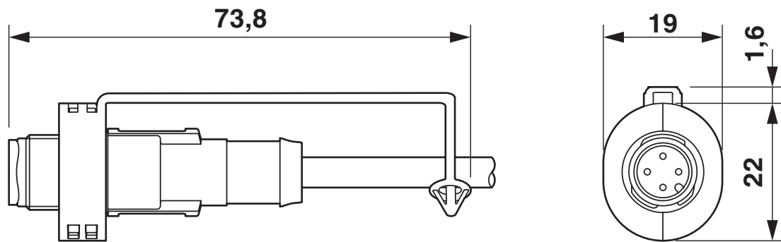
Dessin coté
