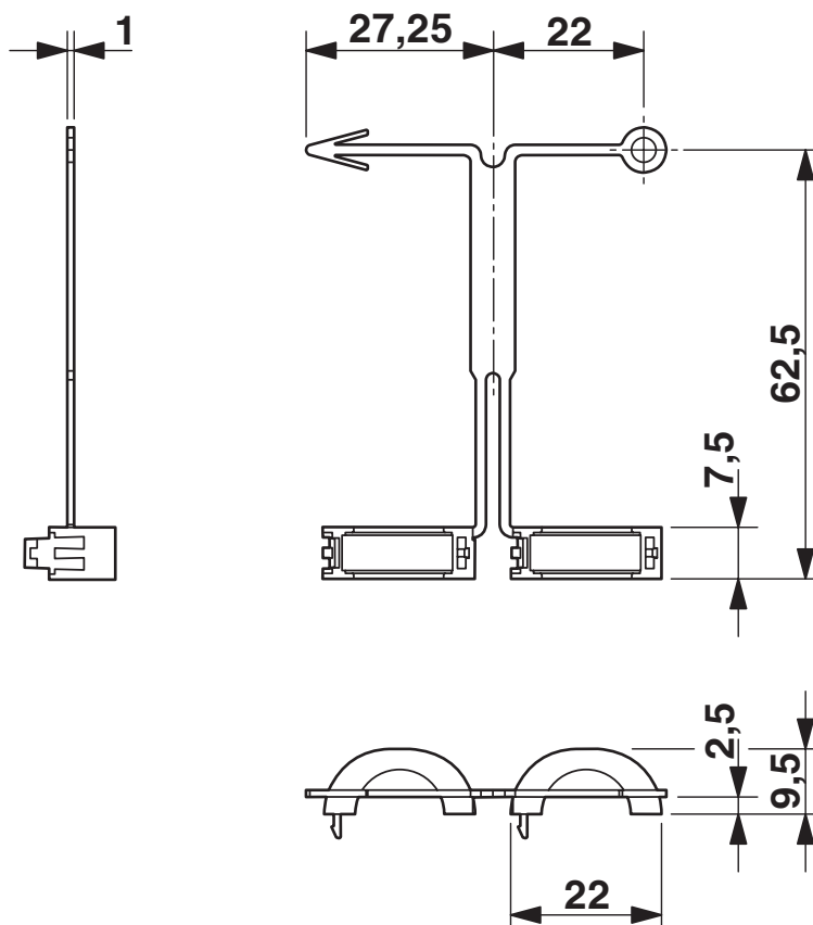
Dessin coté
