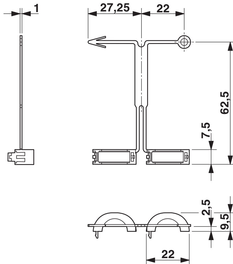
Dessin coté
