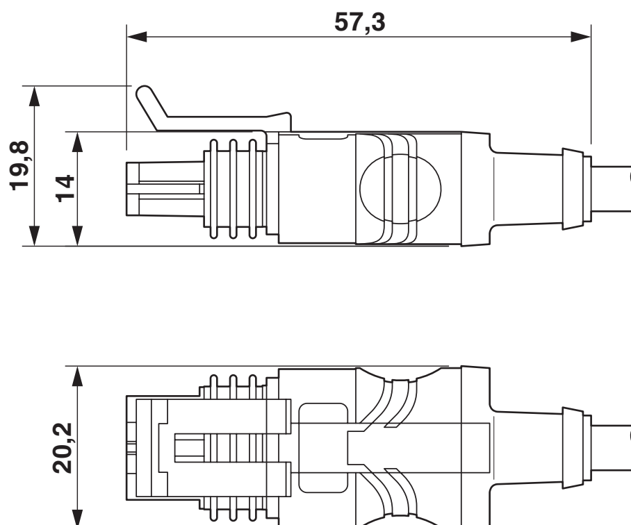
Dessin coté
